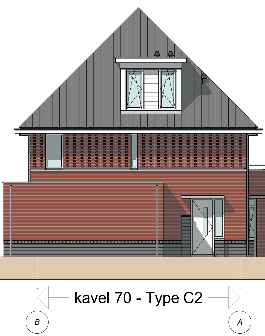
Linkergevel
