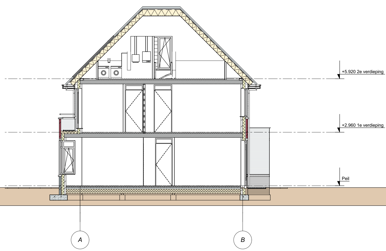
Doorsnede A
