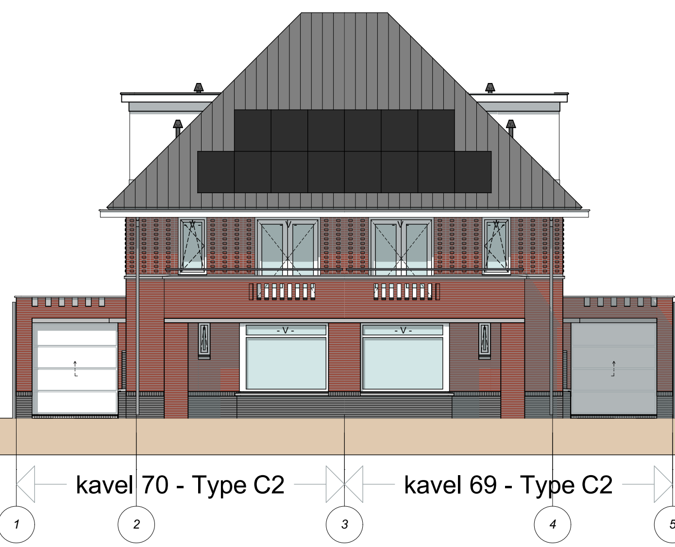
Voorgevel
