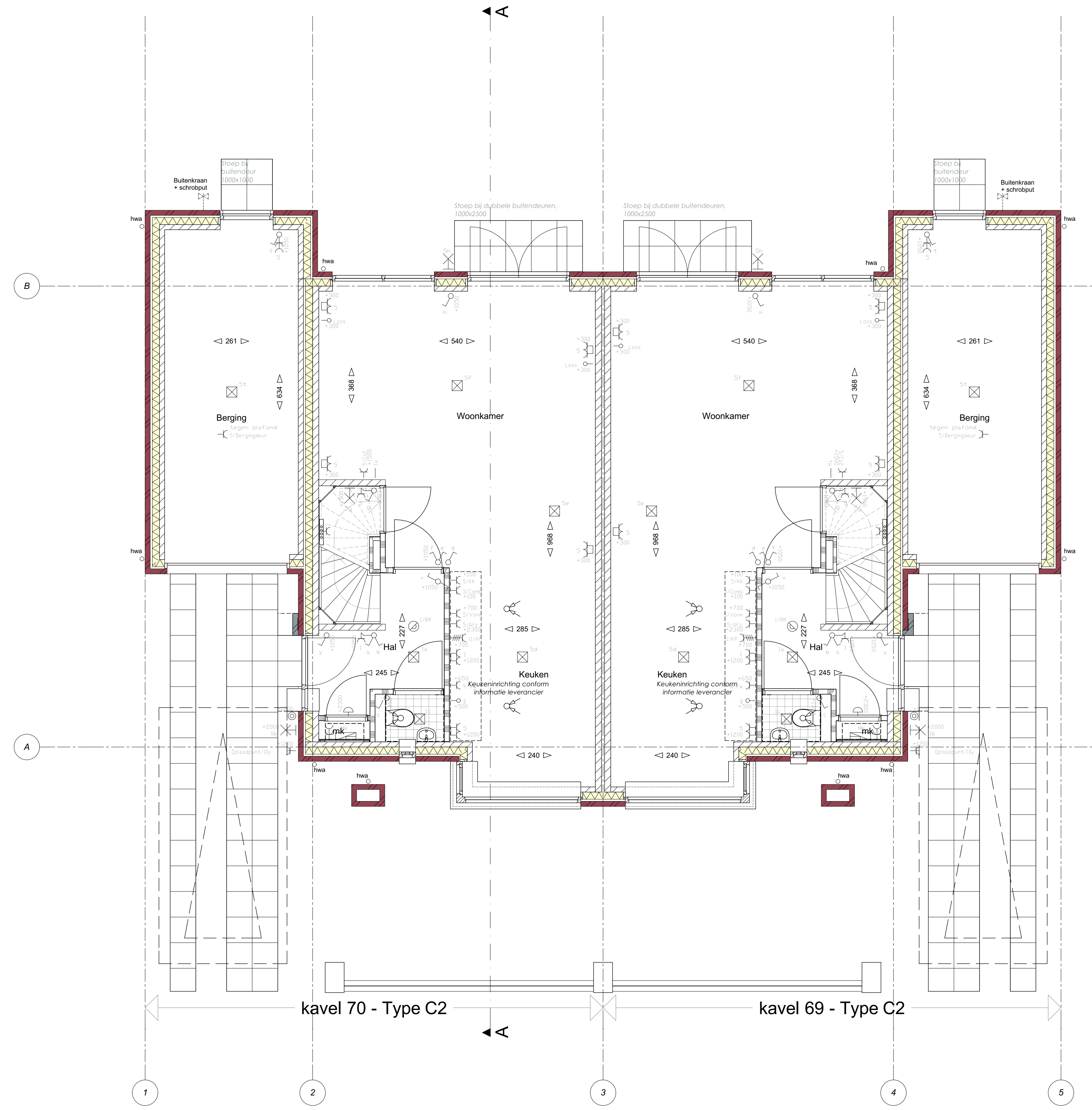
Begane grond
